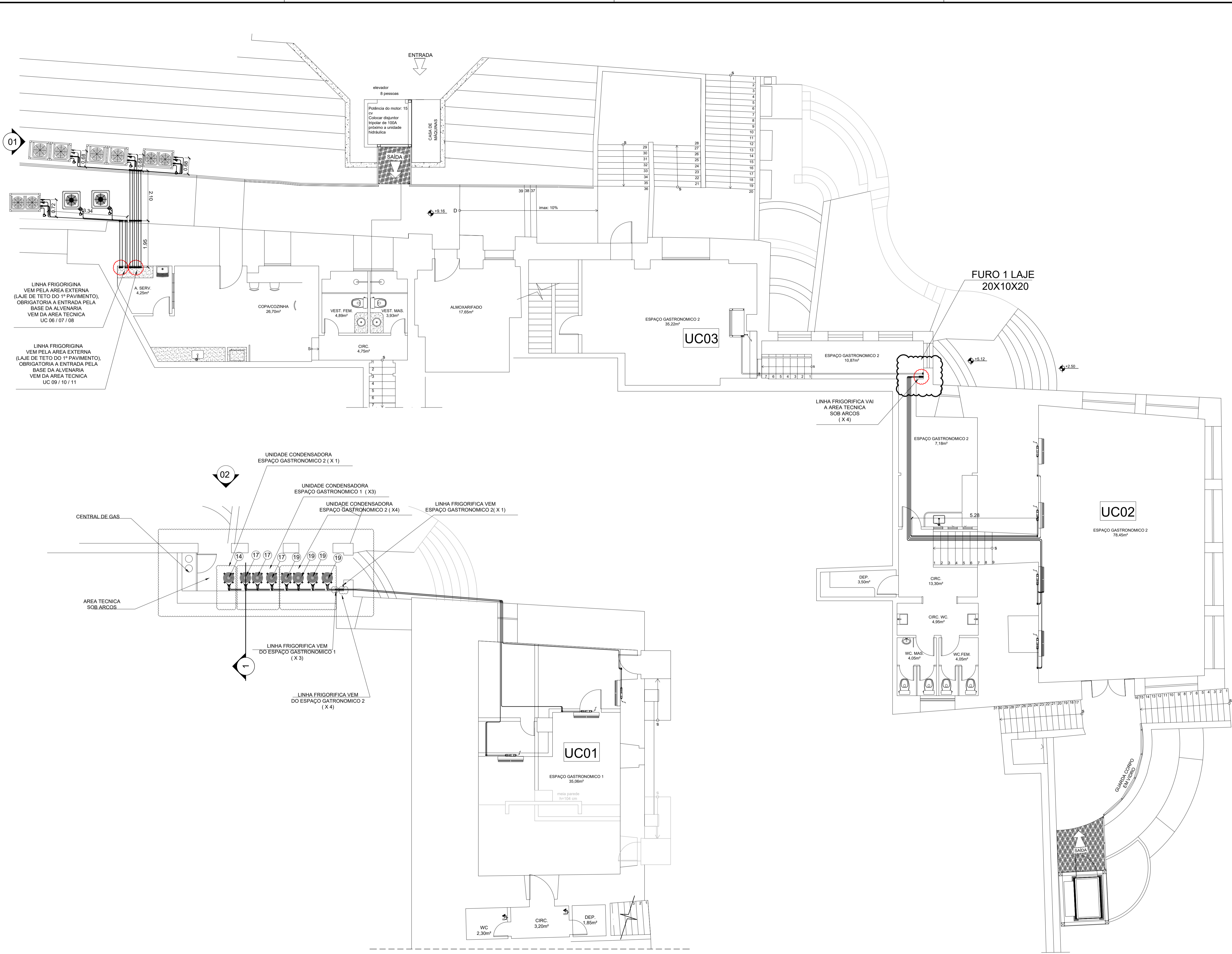
PLANTA BAIXA 1º PAVIMENTO REFORMA DO SALDANHA DA GAMA ESCALA 1/75
