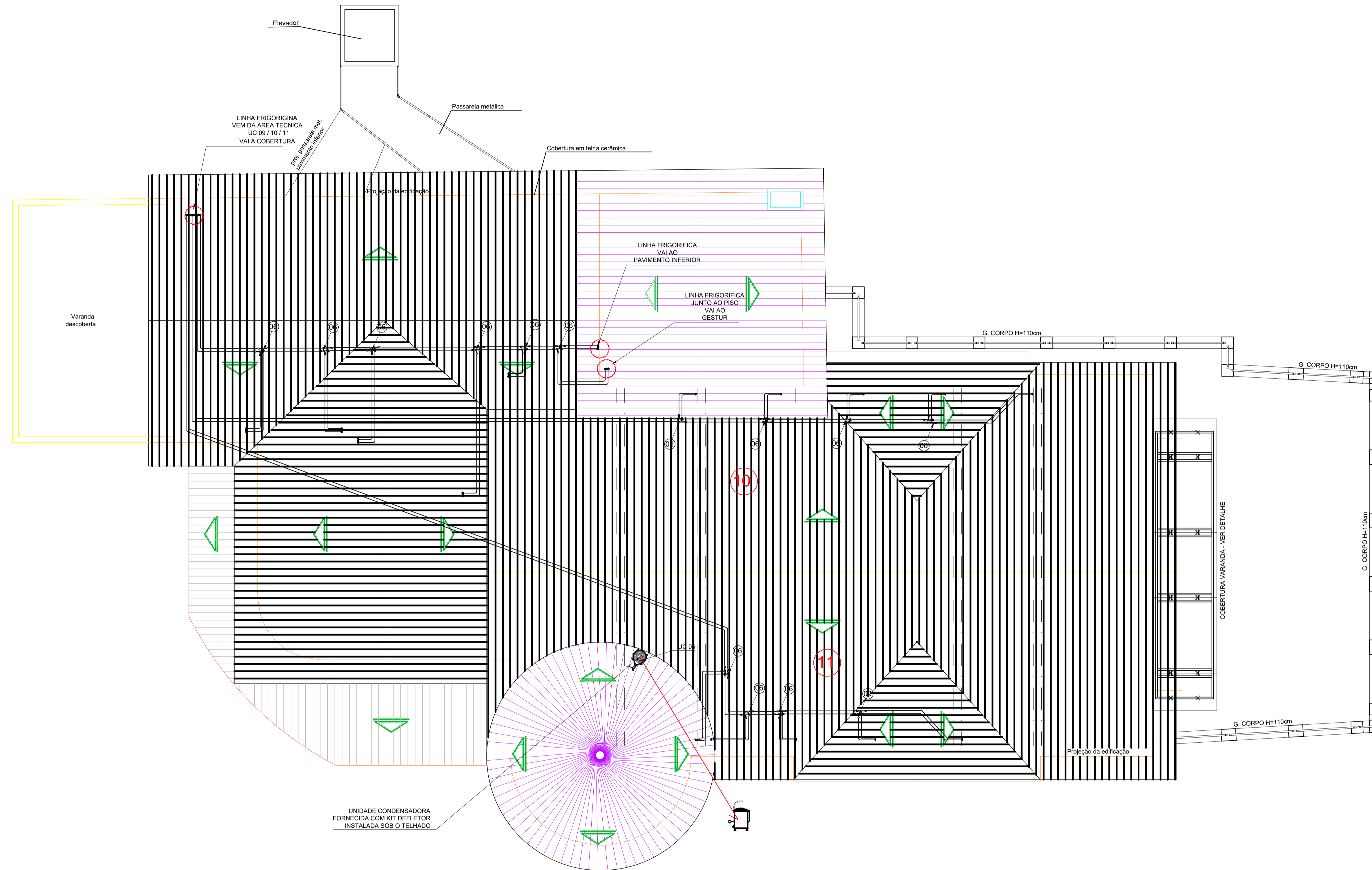
PLANTA BAIXA COBERTURA REFORMA DO SALDANHA DA GAMA ESCALA 1/75
